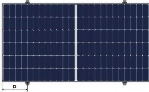
Installation eines gerahmten Moduls mit Befestigungen an den Längsseiten Balken senkrecht zu den Längsseiten (Klemmlänge \geq 50 mm)
